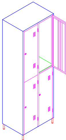
GR-4 Dimensões(mm):628x420x1950 compartmento:300x420x950
