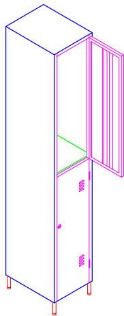
GR-2 Dimensões(mm):328x420x1950 compartmento:300x420x950
