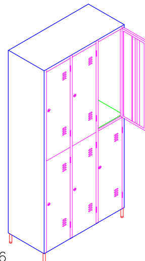
GR-6 Dimensões(mm):928x420x1950 compartmento:300x420x920
