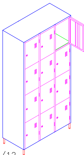
GR-6/12 Dimensões(mm):928x420x1950 compartmento:300x420x460
