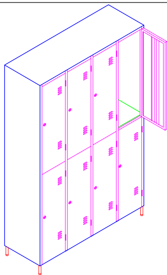
GR-8 Dimensões(mm):1228x420x1950 compartmento:300x420x920
