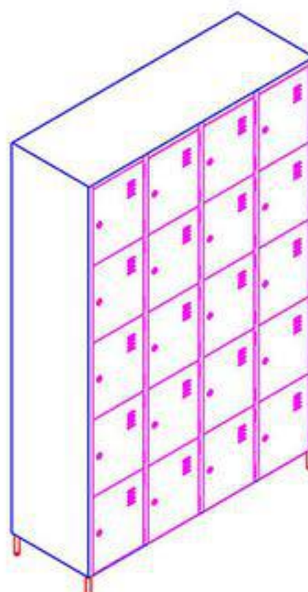
GR-20 Dimensões (mm): 1228x420x1950 Compartimento: 300x420x370
