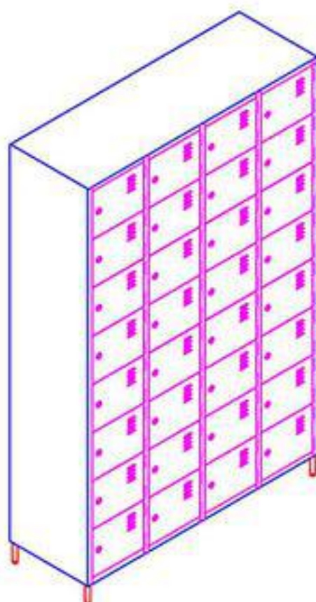
GR-32 Dimensões (mm): 1228x420x1950 Compartimento: 300x420x230
