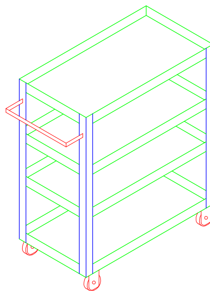
MOD. CSL4 RODIZIOS MÓVEIS DE 3"φ
